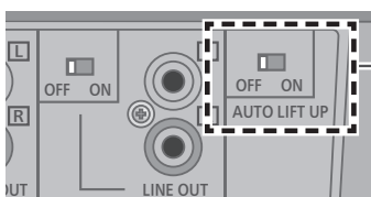
Interrupteur de levage automatique
